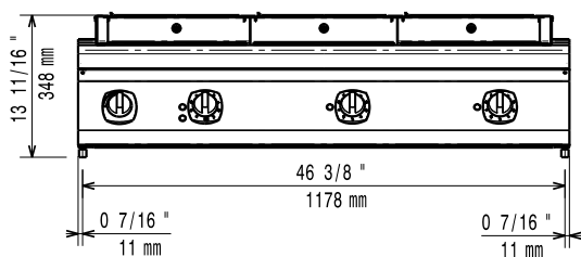
Előlnézet
