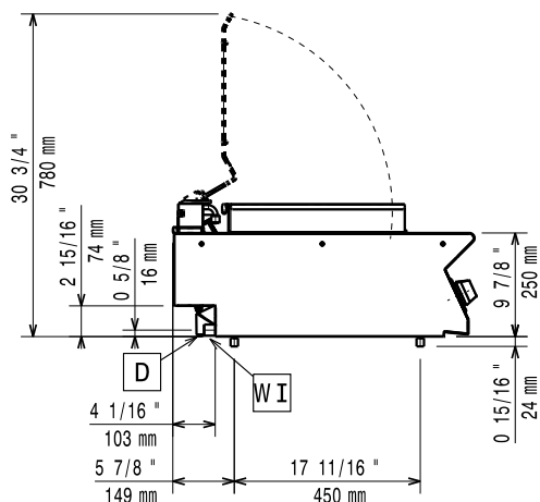
Oldalnézet
