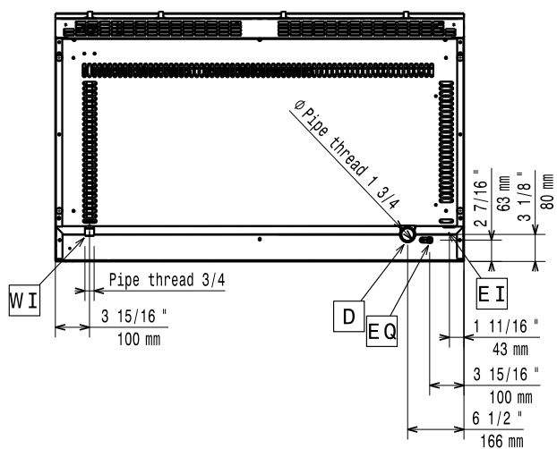
Felülnézet
